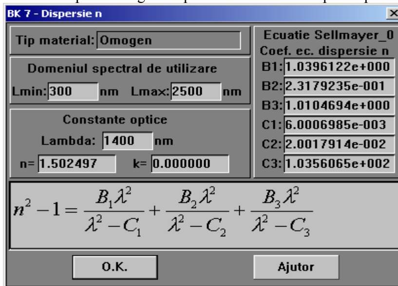
Fig. 11 Fereastra pentru editat coef. ecuatiei de dispersie pentru n.
